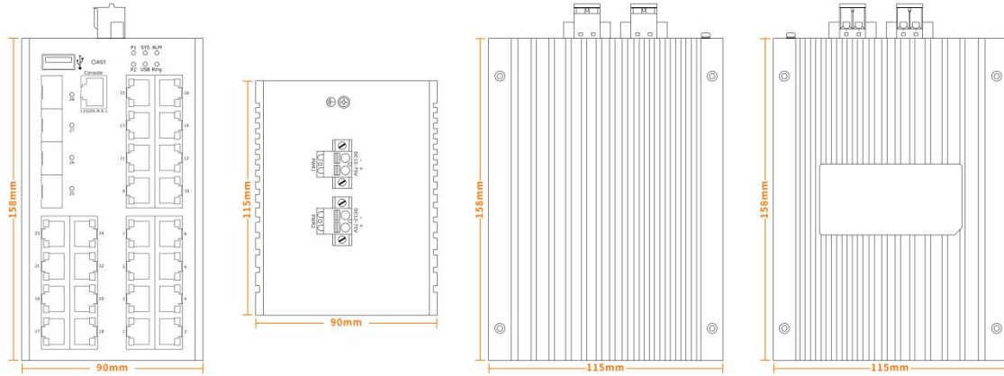
LT-IS6328XG-4XS24GT-D
