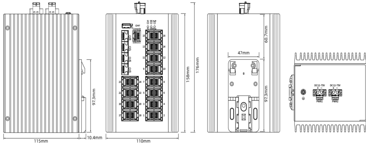
LT-IS6328G-4GX24GT
